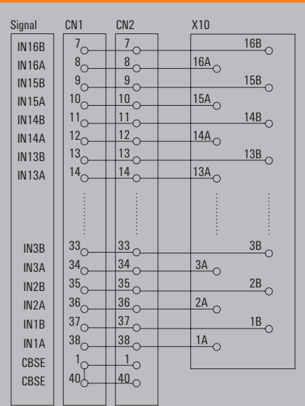
Schematic 1371150000/1371170000 (SAI143)
