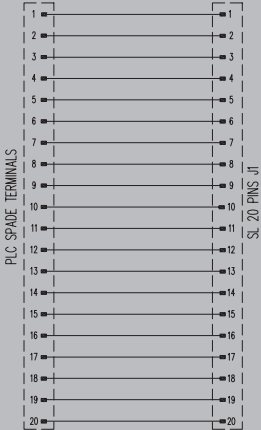
FAD S5135 SL20 R
